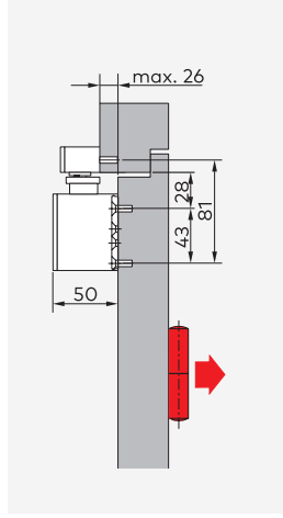
Kapı kanadına itme yönünde montaj TS 92 XEA G Yaklaşık 120°-145° açılma olanağı sağlar.
