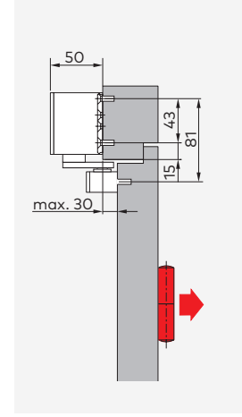
Kapı kanadına itme yönünde montaj TS 92 XEA B Yaklaşık 120°-145° açılma olanağı sağlar.
