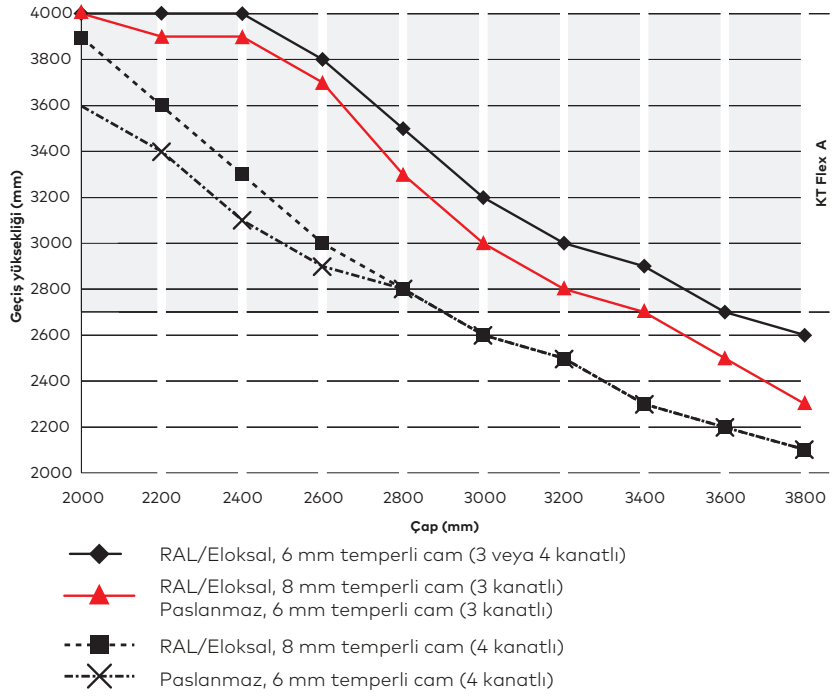
KT Flex 3/4 standart kanat için çap/yükseklik tablosu
