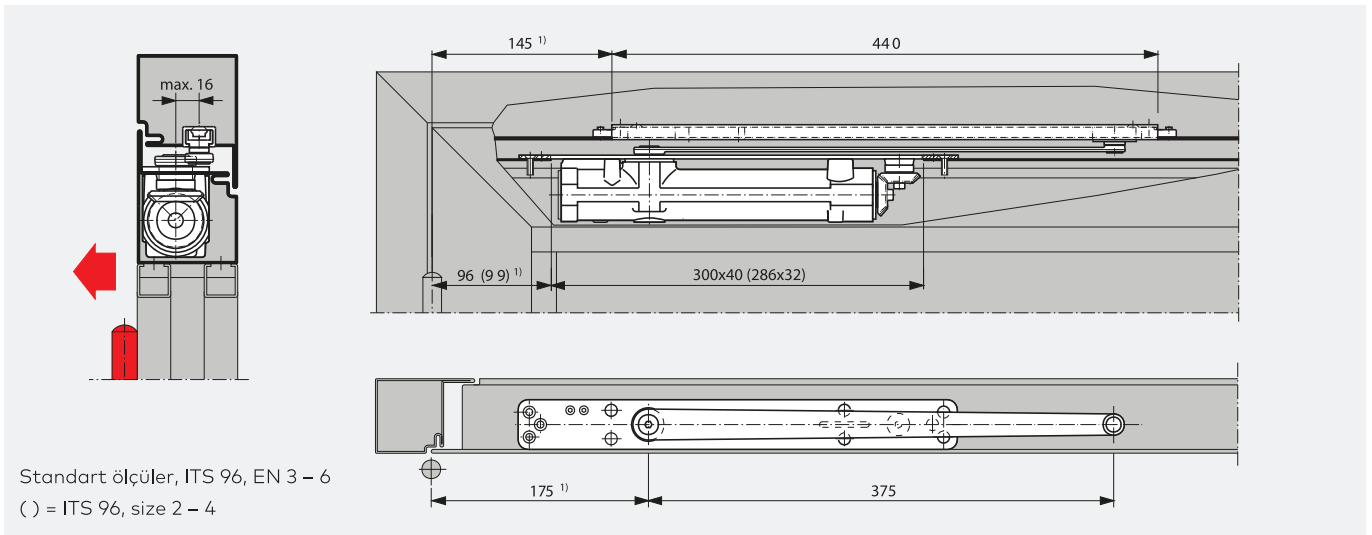
ITS 96 alüminyum kapı uygulaması
