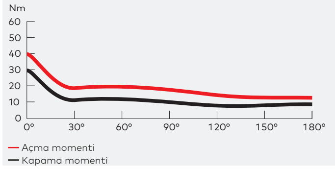
Kapı kanadına çekme yönünde montaj TS 92 XEA B Yaklaşık 180° açılma olanağı sağlar.
