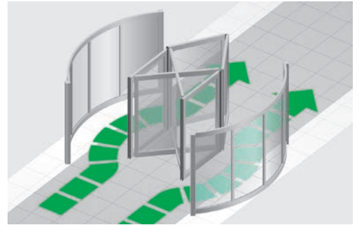
KTC-4, panik kaçış pozisyonu
