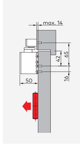
Kapı kanadına çekme yönünde montaj TS 92 XEA B Yaklaşık 180° açılma olanağı sağlar.
