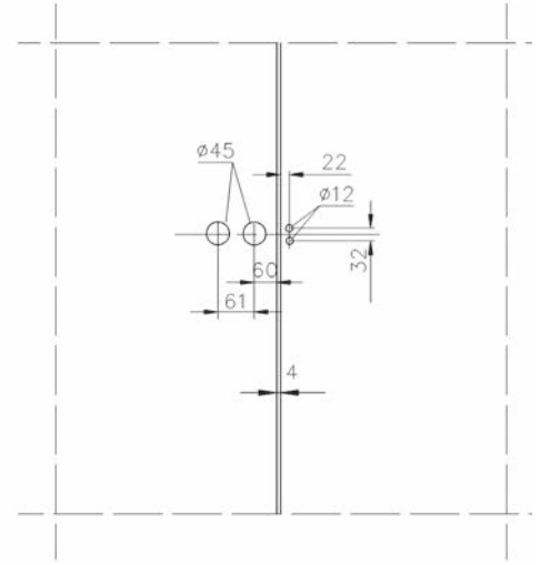
Arcos Studio cam cama kilit karşılığı cam delik detayı
