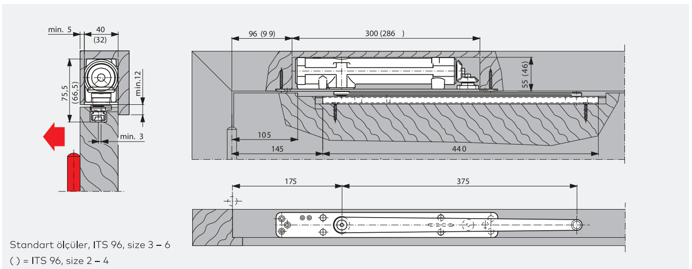
ITS 96 ahşap kapı uygulaması
