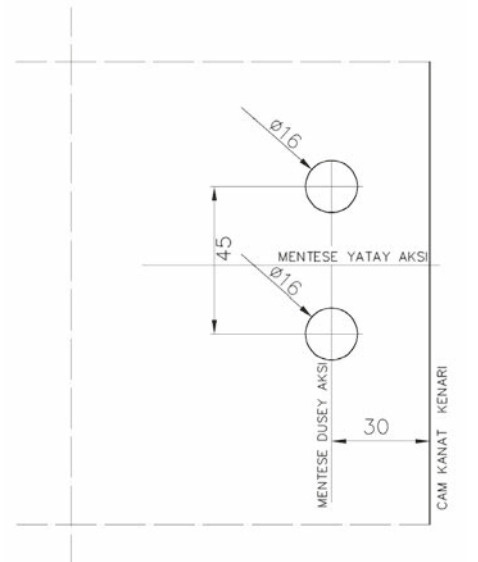
Junior Office yaprak menteşe cam delik detayı
