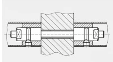
MIM-432-00-052 GZ 214 (28-75 mm) Ahşap/metal kapılar için çift tarafli bağlantı elemanı
