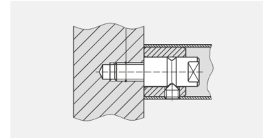
MIM-432-00-121 GZ 234 Çerçevesi kapılar için (20mm vida derinliği) Tek tarafli bağlantı elemanı
