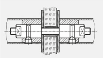
MIM-432-00-047 GZ 215 (8-15 mm) Cam kapılar için çift tarafli bağlantı elemanı
