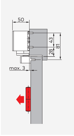
Kapı kanadına çekme yönünde montaj TS 92 XEA G Yaklaşık 180° açılma olanağı sağlar.
